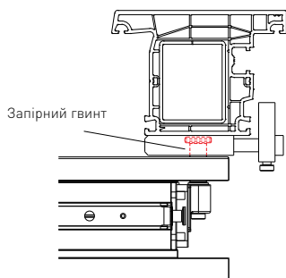
17202-00-N03 Шаблон для бокової запірної пластини
