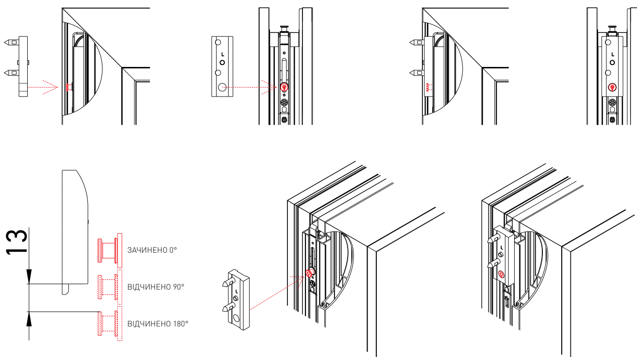
I7203-00-N03 Маркувальний шаблон для запірних пластин
