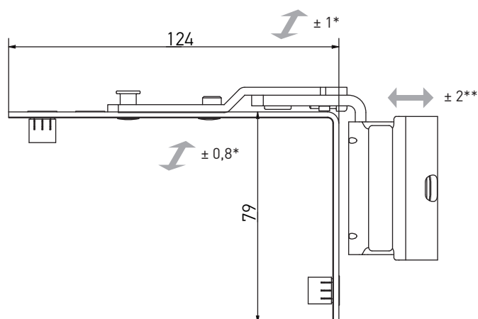
Ножиці поворотні
