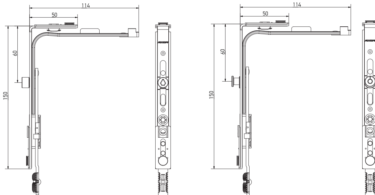
Кутова передача вузька, 1 ML, 50x150
