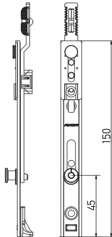
Поворотний шпінгалет 90° (нижній), 1 MR
