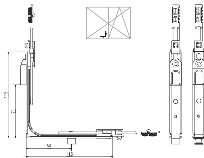
Кутова передача для штупльової стулки, 1 ML, 115×115, нижня
