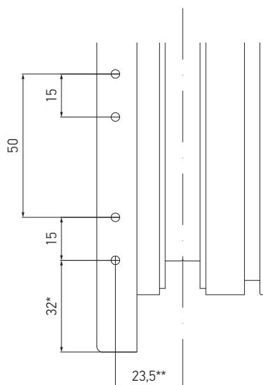
Вісь паза фурнітури
