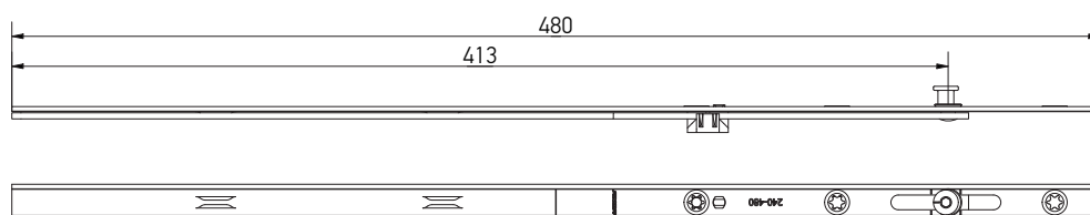
Лінійний подовжувач 480 мм з можливістю підрізки, 1 MR
