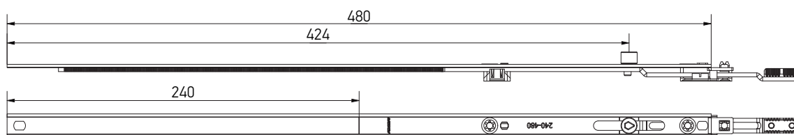
Лінійний подовжувач 480 мм, 1 ML
