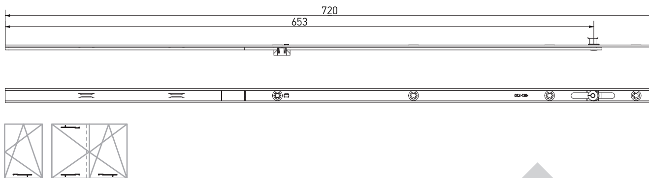
Лінійний подовжувач 720 мм з можливістю підрізки, 1 MR
