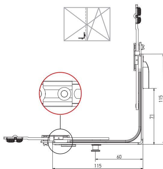
Кутова передача для штупльової стулки, 1 MR, 115×115, нижня
