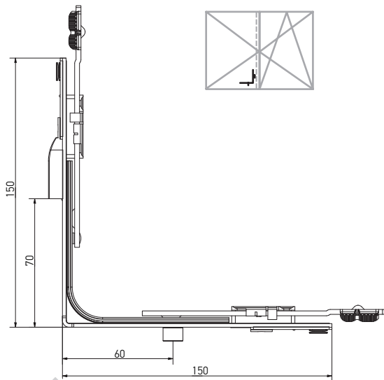
Кутова передача для штульпової ступки, 1 ML, 150×150, нижня
