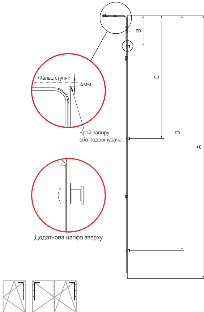
Середній запір з додатковою цапфою, MR
