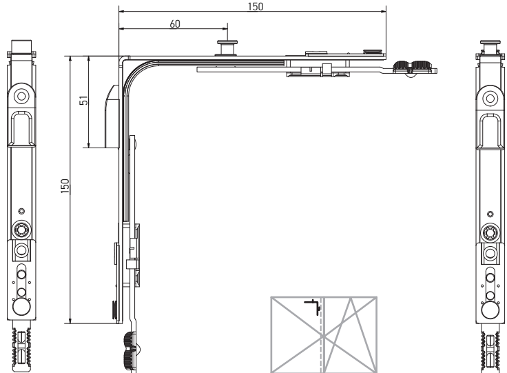
Кутова передача для штульпової ступки, 1 MR, 150×150, нижня
