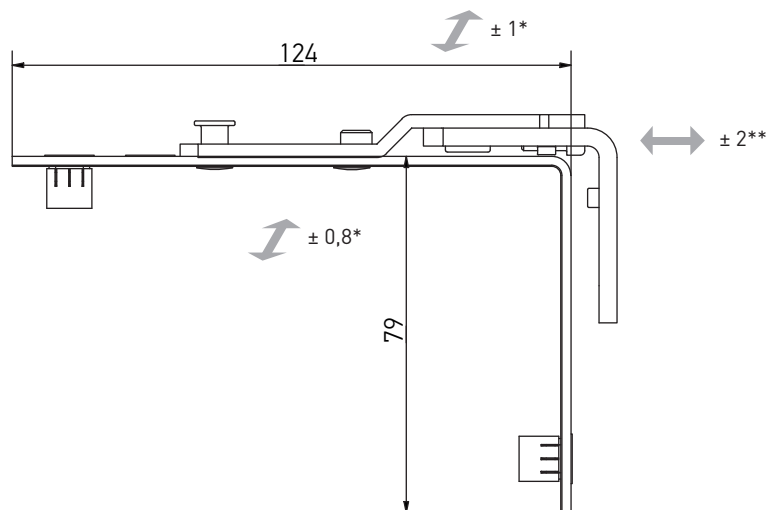
Ножиці поворотні
