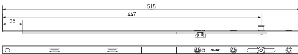
Лінійний подовжувач з можливістю підрізки, 1 MR
