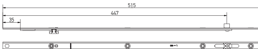
Лінійний подовжувач для кутової передачі 480 мм, 1 ML
