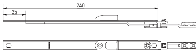
Подовжувач для штільової стулки 240 мм
