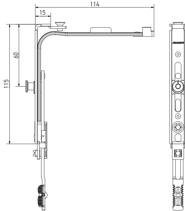
Кутова передача вузька, 1 MR, 115x15
